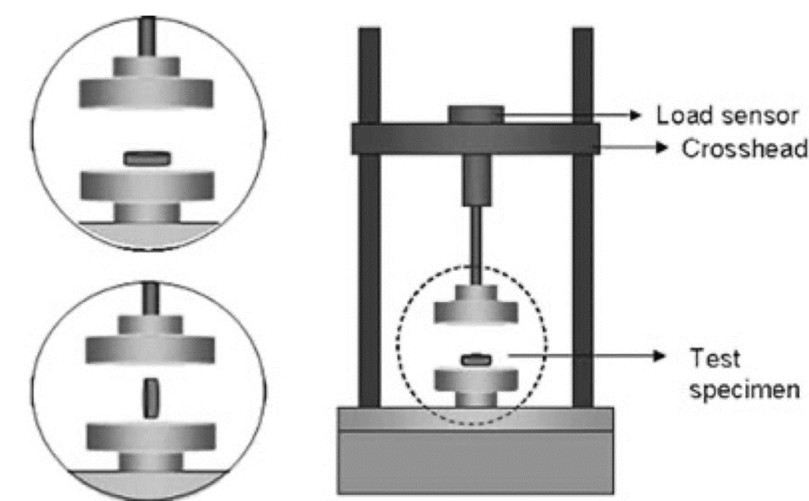
Figura 1. Máquina de Testes Universal [6]
